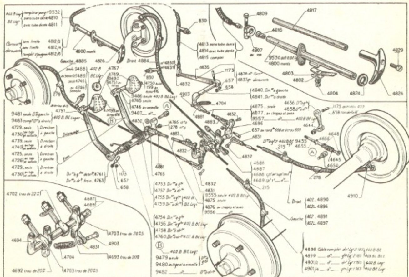
402 B. — Mécanisme de Freins
