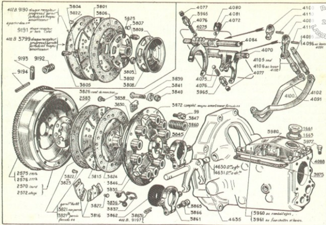
402 B. - Embayage
