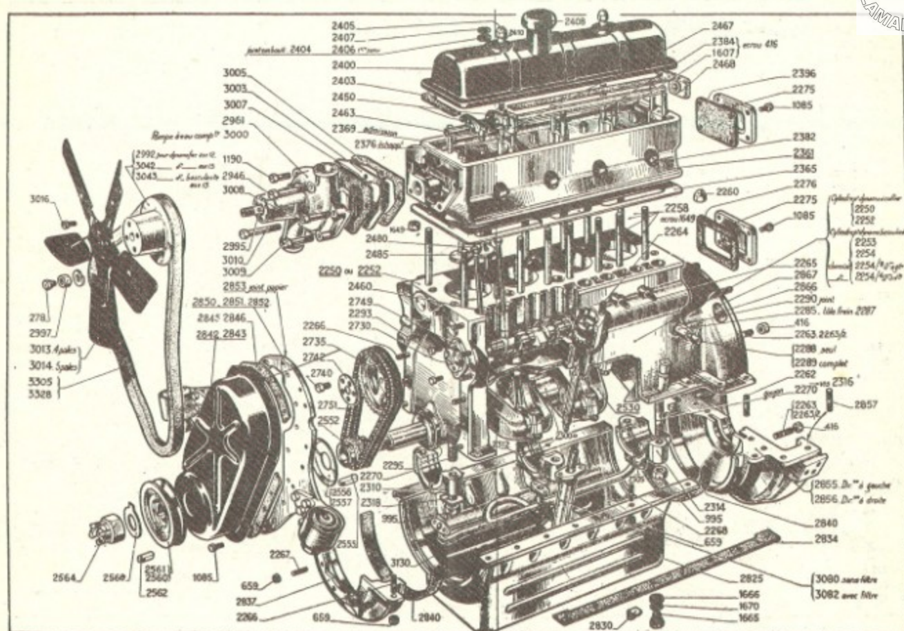
402. - Moteur
