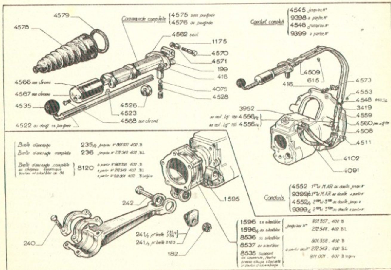
402 B. — Changement de Vitesses
