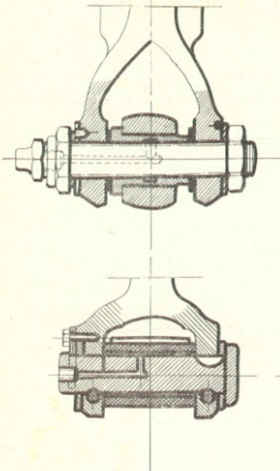
Fig. 1. — Articulation de la tête d'essieu
