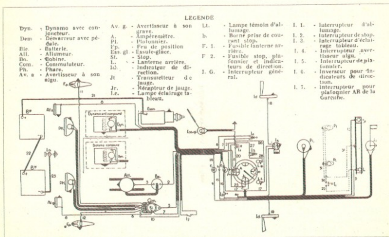
Schéma de l'équipement électrique
