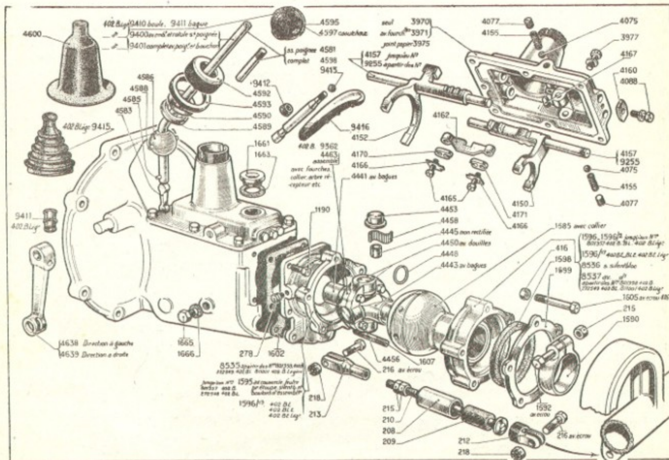
402 B. — Commande par leviers, couvercle, rofules, support de poussée
