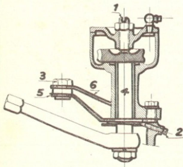
Fig. 2. — Réglage de la direction
